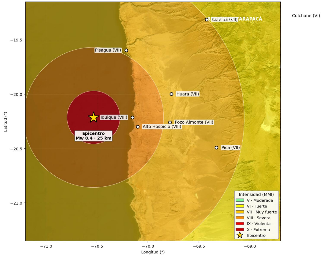
(Imagen 1) — ShakeMap referencial: intensidad de sacudida (MMI) estimada para el escenario ficticio (Mw 8,4, 40 km al W de Iquique, 25 km de profundidad). Modelo de atenuación de intensidad tipo IPE; estimación con fines exclusivamente docentes.
